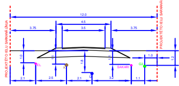
PROJEKTĒTĀS IELAS ŠĶĒRSPROFĪLS B - B
